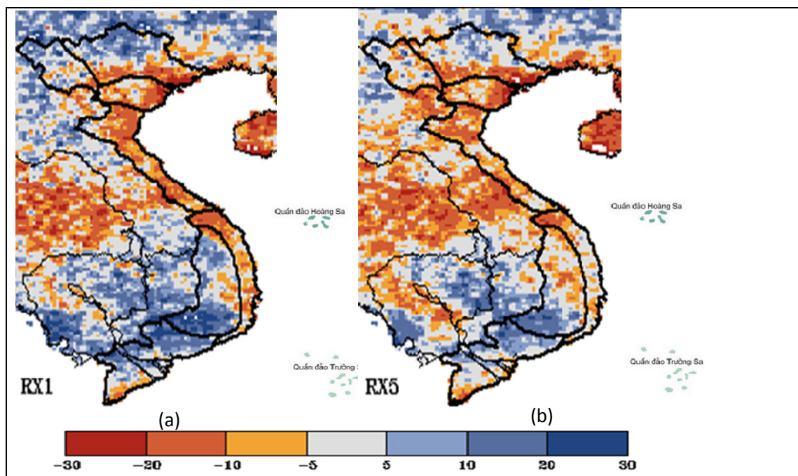
Hình SPM-7. Dự tính biến đổi lượng mưa 1 ngày lớn nhất (a), 5 ngày lớn nhất (b) vào cuối thế kỷ 21 theo kịch bản cao RCP 8.5 (%)
