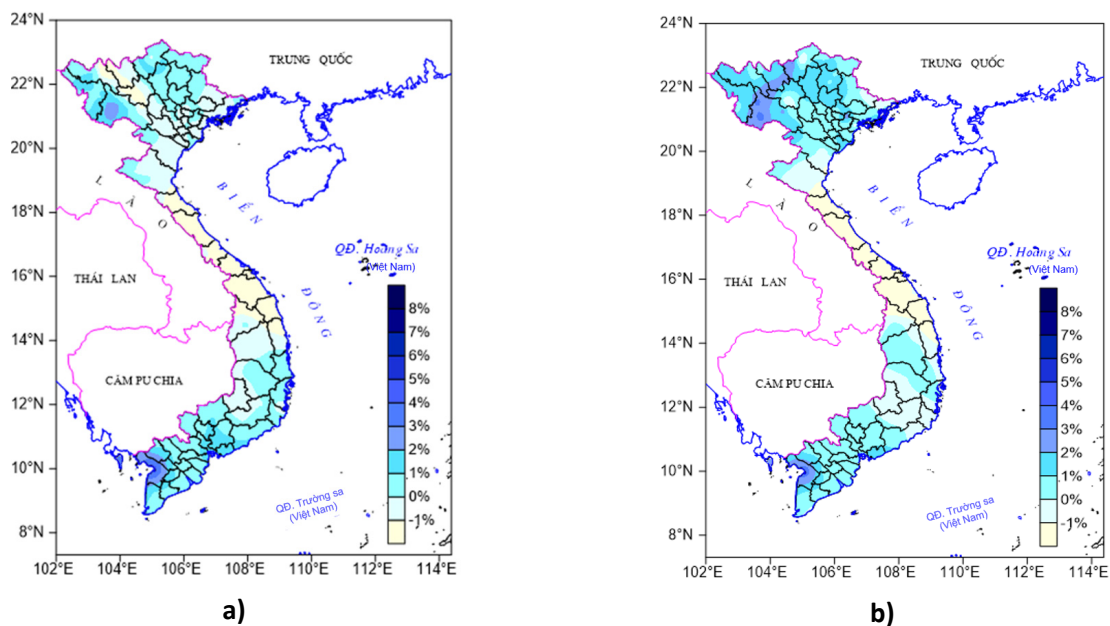
Hình SPM-6. Dự tính biến đổi của số ngày có mưa trên 50 mm vào giữa (a) và cuối (b) thế kỷ 21
