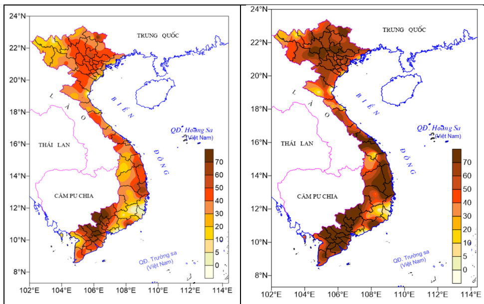
Hình SPM-5. Dự tính biến đổi số ngày nắng nóng thời kỳ giữa (trái) và cuối (phải) thế kỷ 21 so với trung bình thời kỳ 1980-1999 theo kịch bản trung bình
